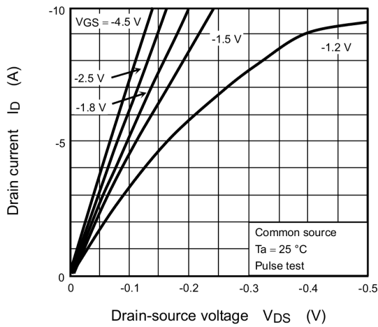
Fig. 7.1 I_D - V_{DS}
